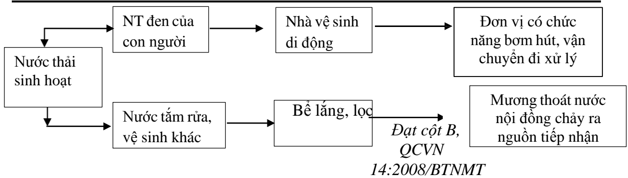
Sơ đồ hệ thống xử lý nước thải sinh hoạt
